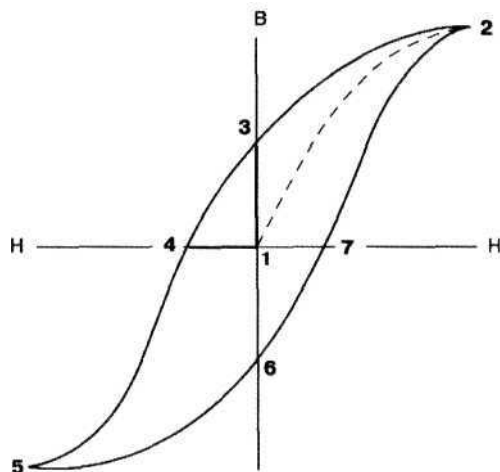
Рис. 4.3.1. Типичная петля гистерезиса для магнитно-твердого ферромагнитного материала. В точке 2 достигается магнитное насыщение. Отрезок 1-3 определяет остаточную магнитную индукцию, а отрезок 1-4 — коэрцитивную силу, характеризующую способность образца противостоять размагничиванию
